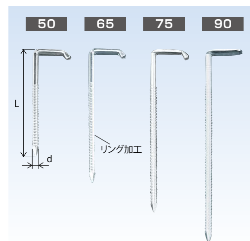
■仕様 【材質】ステンレス SUS304
