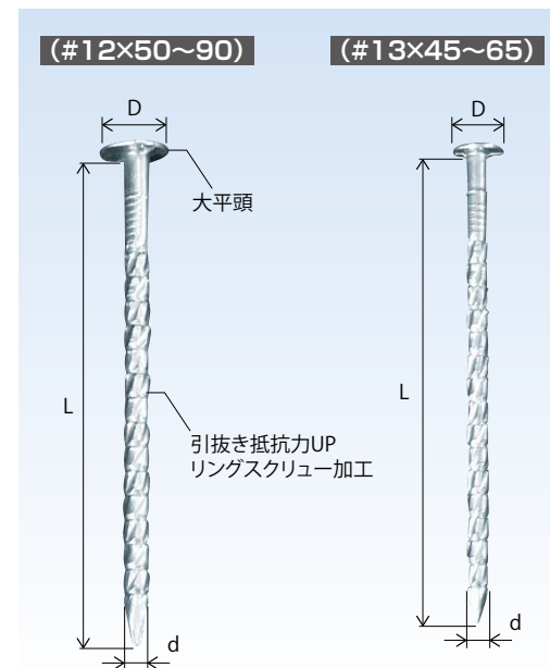
■仕様 【材質】ステンレス SUS304
