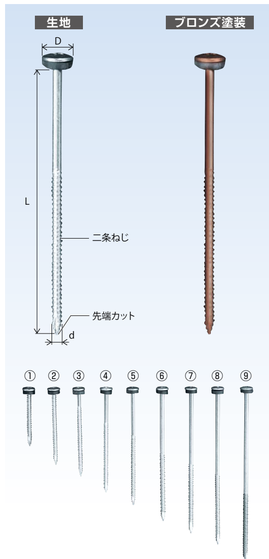
■仕様 生地 【材質】ステンレスSUS305・CRゴムパッキン付
