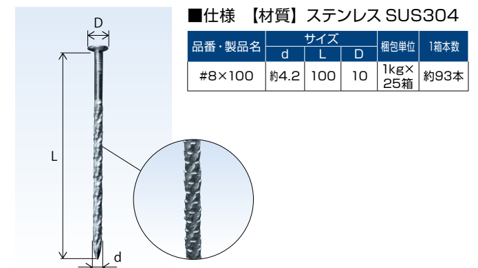
■仕様 【材質】ステンレス SUS304
