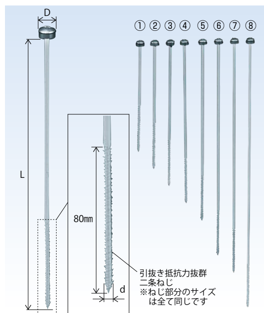
■仕様 生地 【材質】ステンレスSUS305・CRゴムパッキン付
