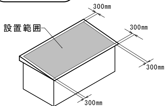
片流の場合
